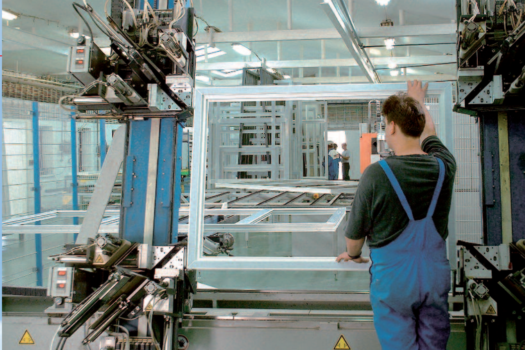
4-hlavový vertikálny zvrací automat - prevádzka Vyšehradné - rok 1998.
